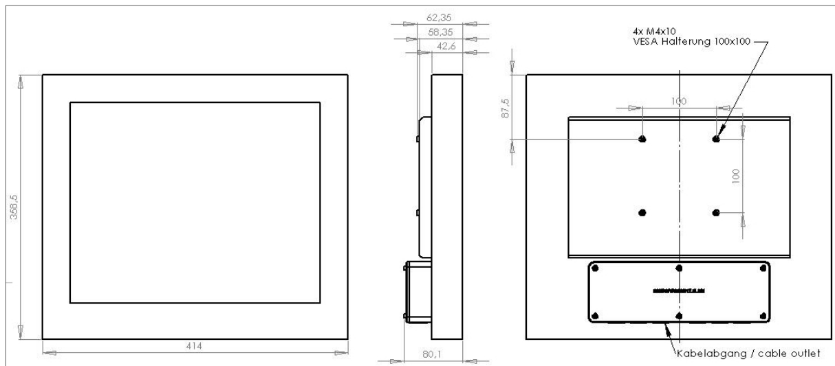
Bild 1: Technische Zeichnung / technical drawing
