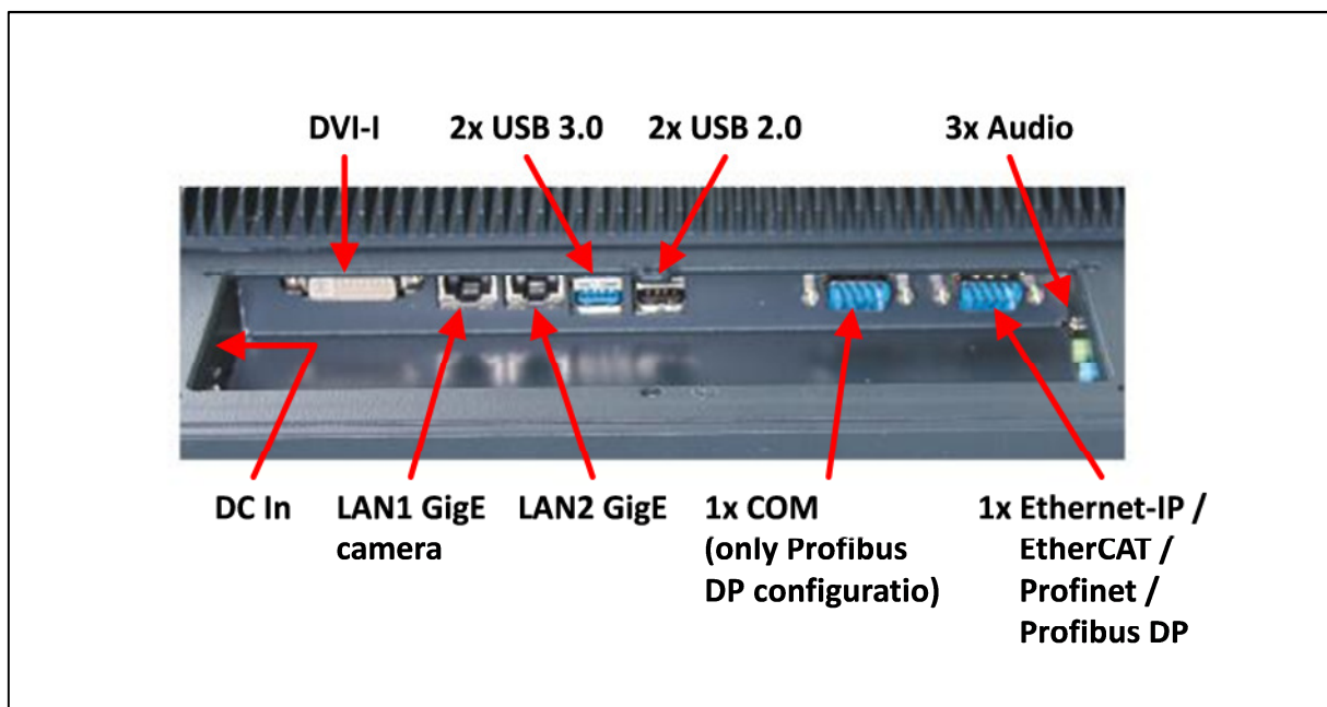
Bild 2: Schnittstellen Rückseite der Profibus-DP-Konfiguration / rear I/O panel Profibus DP configuration
